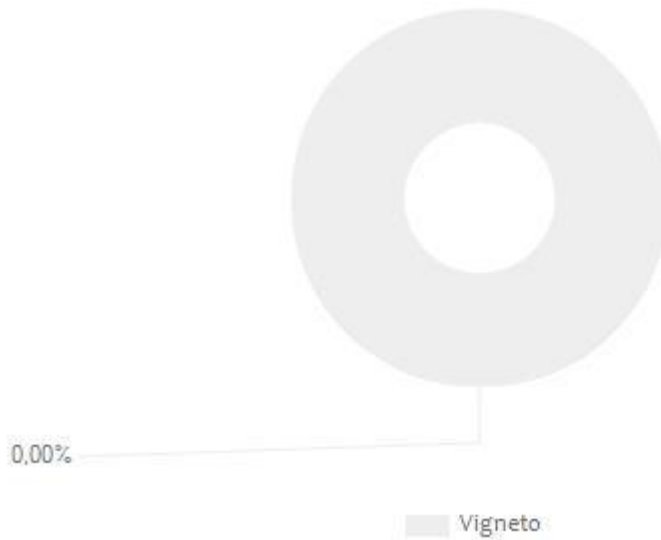
Figura 1. Valori percentuali dei diversi contributi rispetto a “Direct Water Scarcity Footprint” e “Non-Comprehensive Direct Water Degradation Footprint” TOTALI, per una bottiglia di Brunello Riserva .
